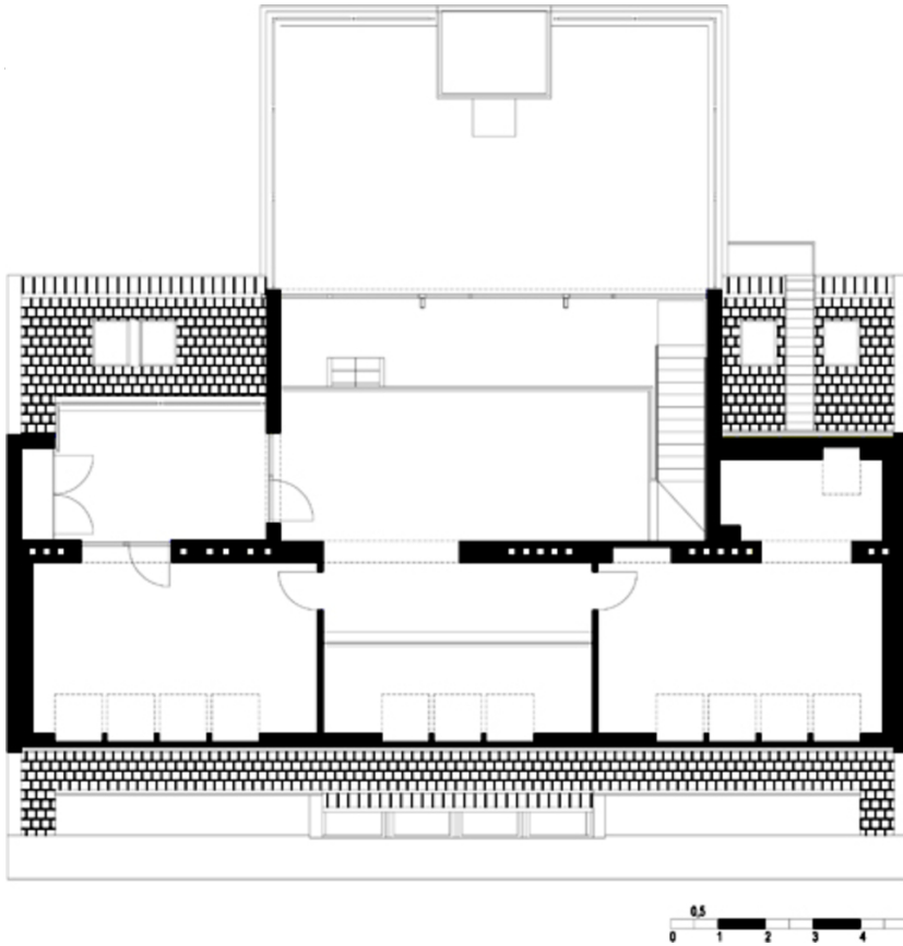
Grundriss DG2
