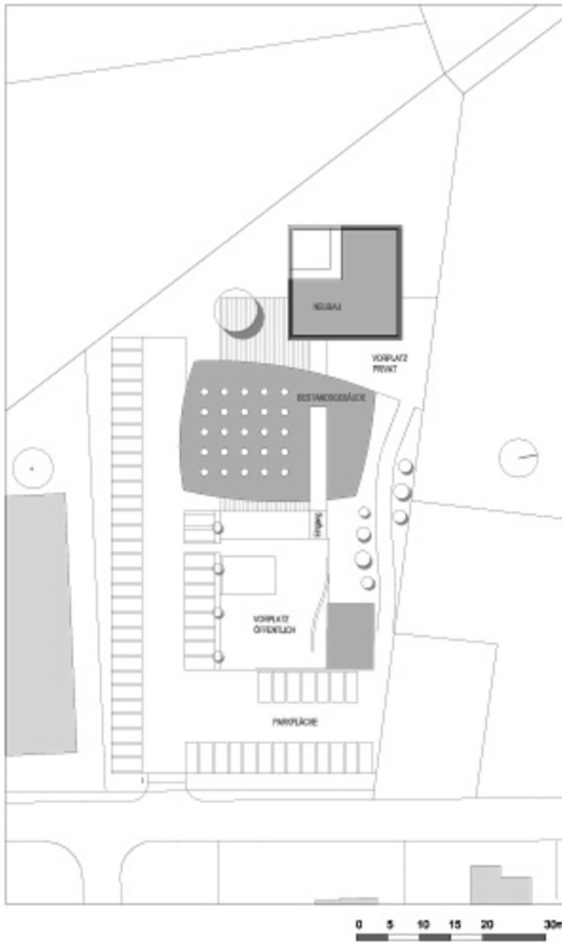
Lageplan
