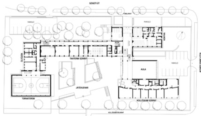
FÖLDSZINTIALAPRAJZ M 1:500
