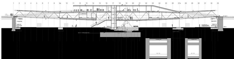
Schiffsstation Längsschnitt
