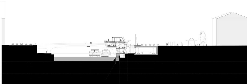
Schiffsstation Querschnitt
