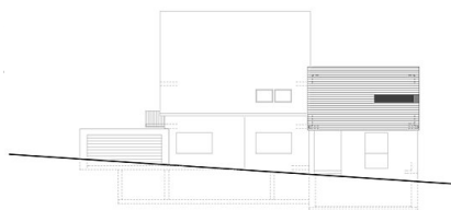
ANSICHT SÜD OST
