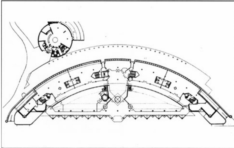
Grundriss EG
