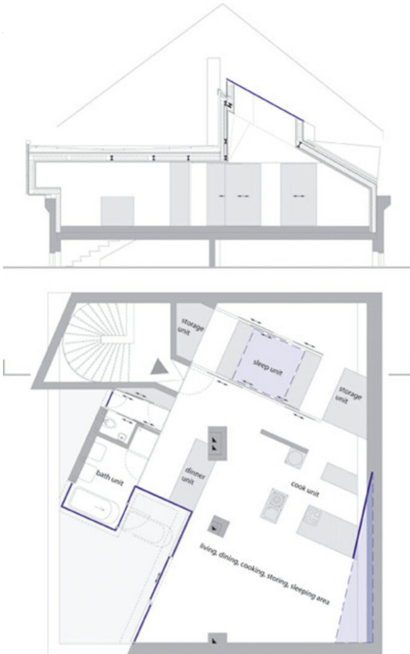
Projektplan
