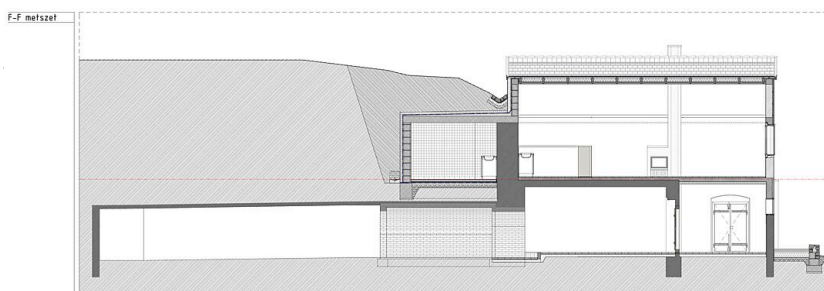
longitudinal section
