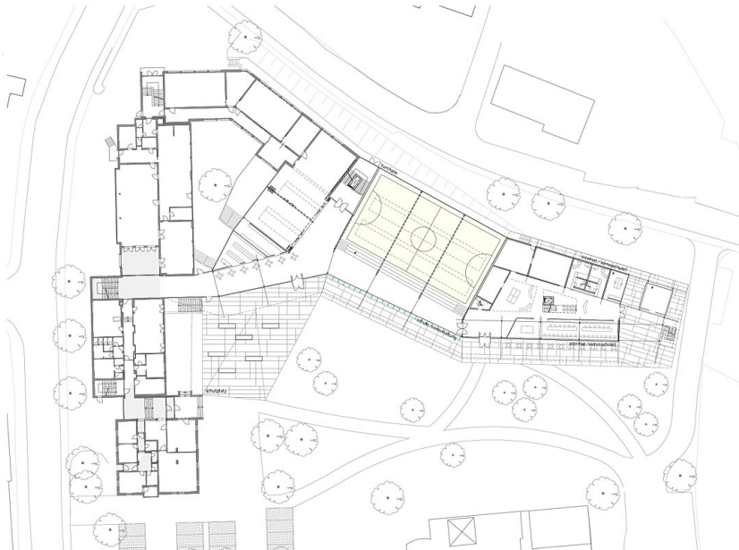
Erdgeschoß + Außenanlagen
