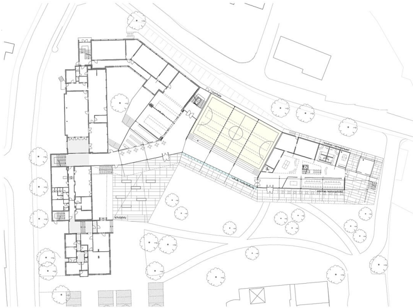
Erdgeschoß + Außenanlagen
