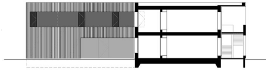
Schnittansicht GRUPPEN
