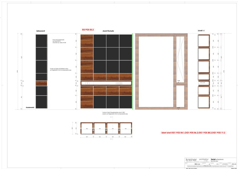
Möblierung
