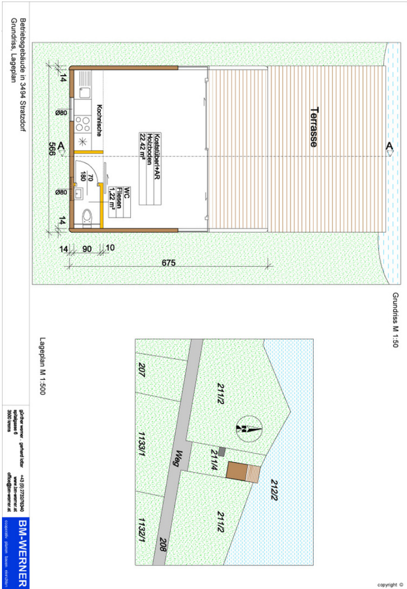
Lageplan
