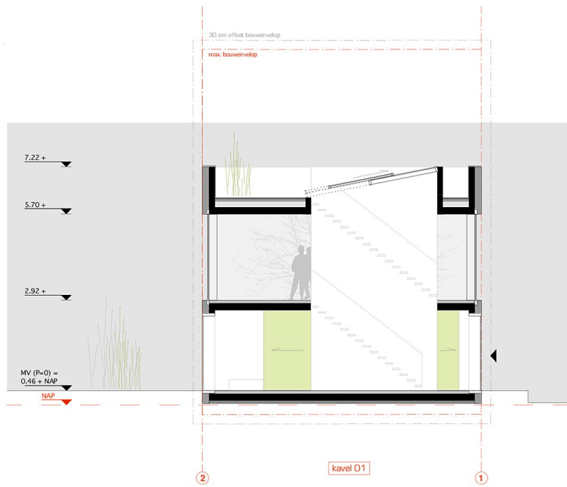
Längsschnitt
