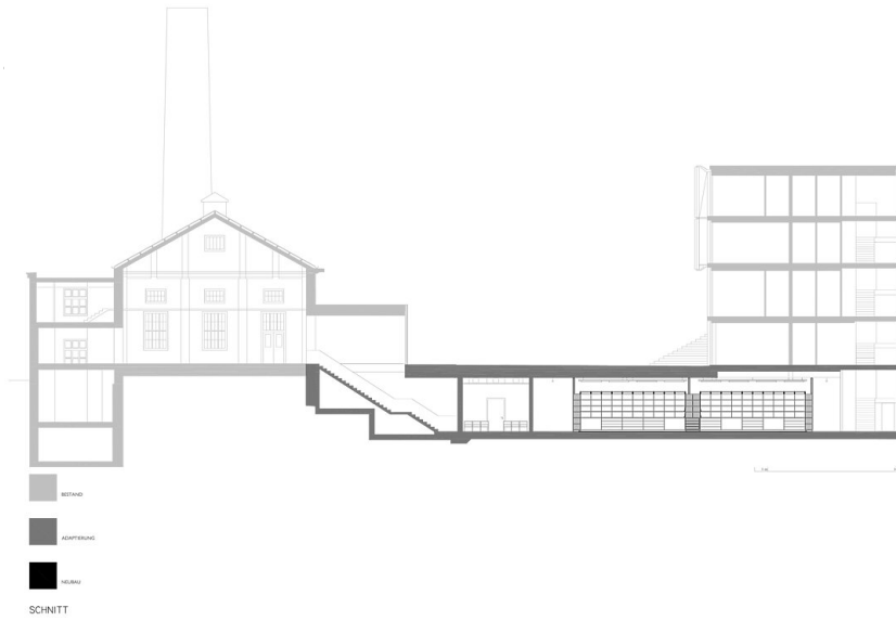
Kesselhaus, Schnitt
