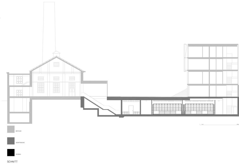
Kesselhaus, Schnitt
