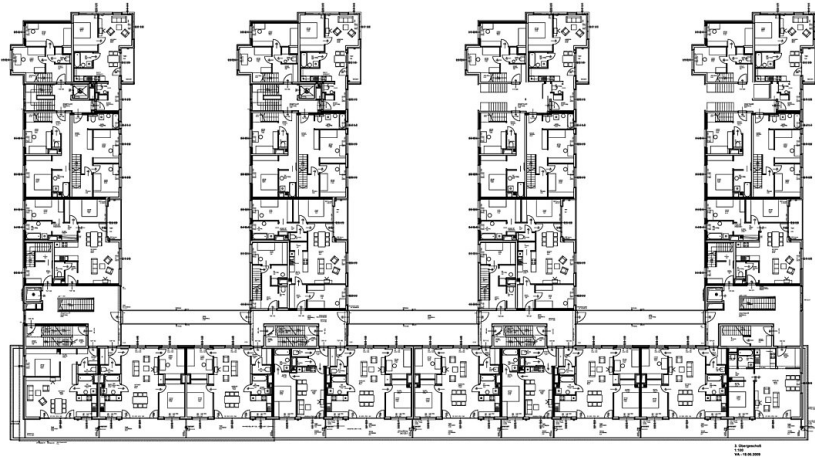
Grundriss 3.OG
