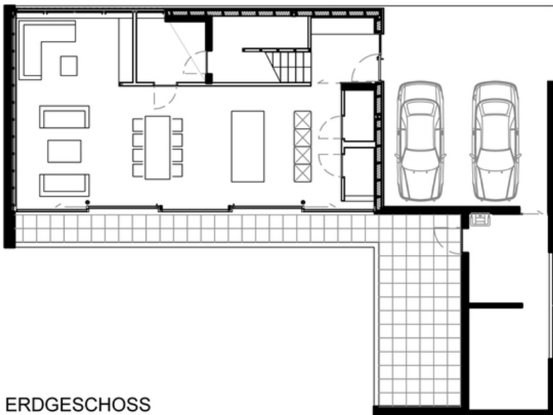
Projektplan
