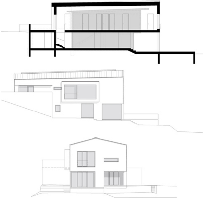
Schnitt, Ansicht
