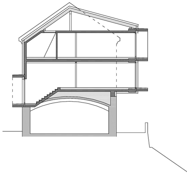
Schnitt 1
