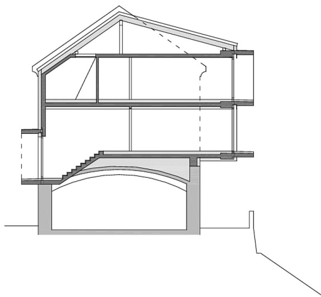
Schnitt 1
