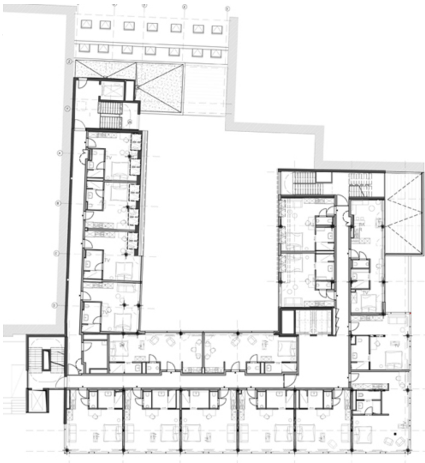
Grundriss OG7
