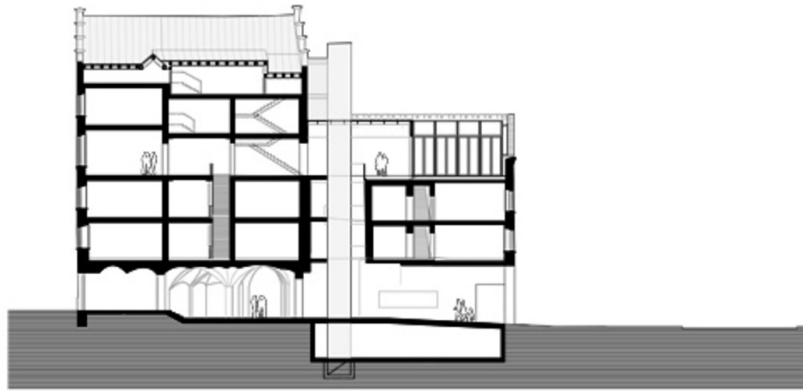
LANGSSCHNITT
