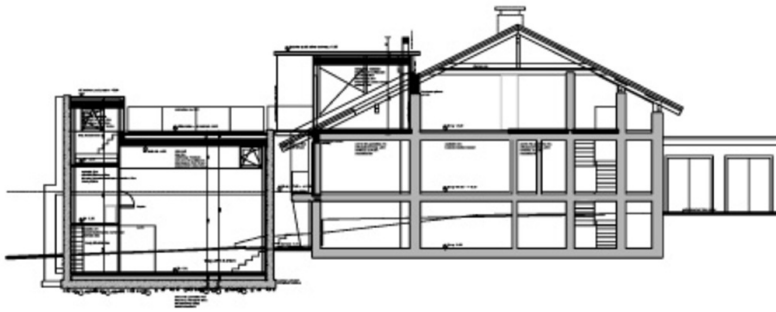
schnitt 1-1
