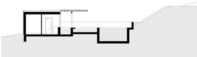
Schnitt 1
