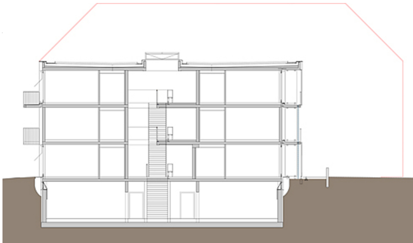
Schnitte
