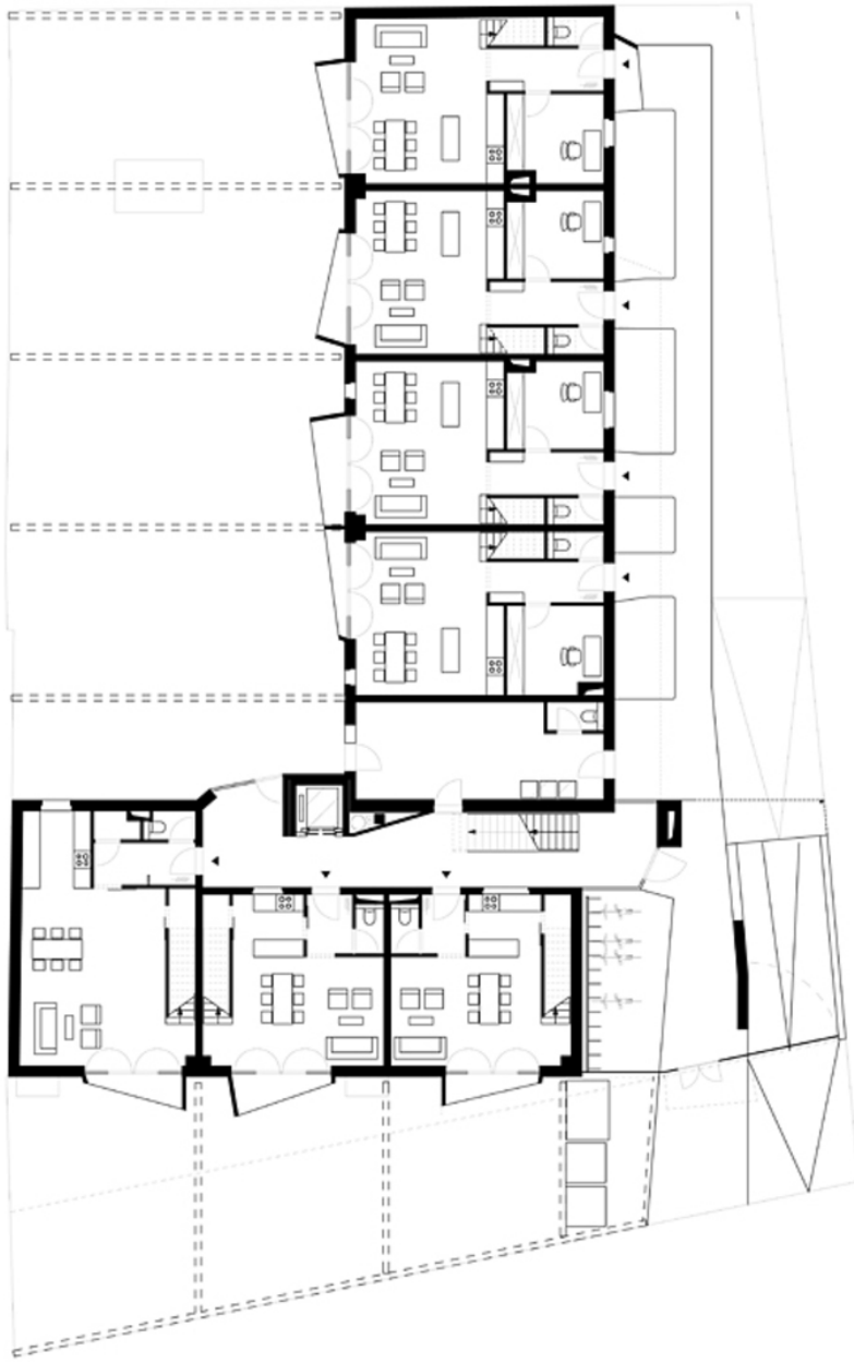
Grundriss EG
