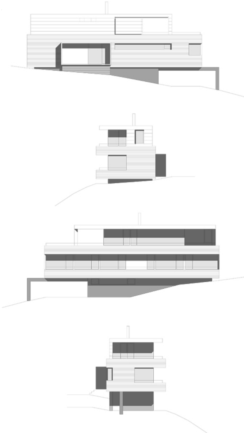
Ansichten
