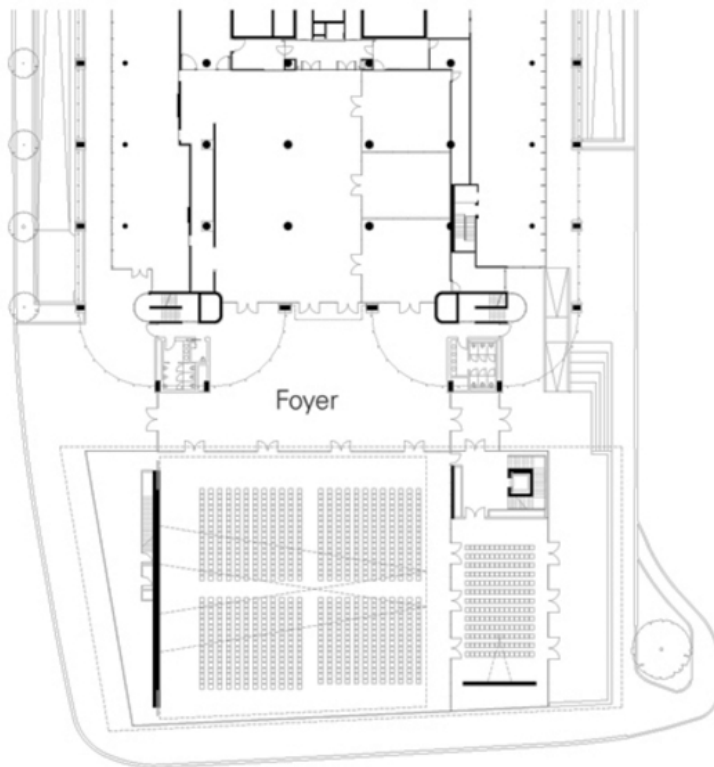
Grundriss Erdgeschoss 1:1000
