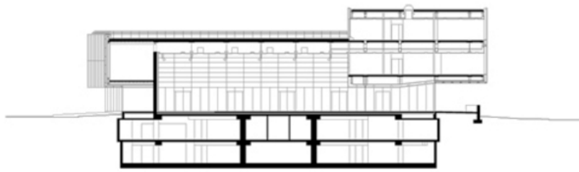
Schnitt 1:1000
