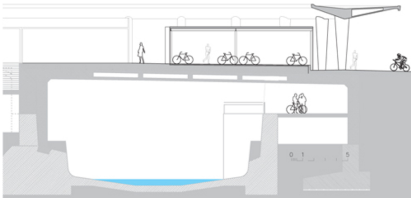
Schnitt 1
