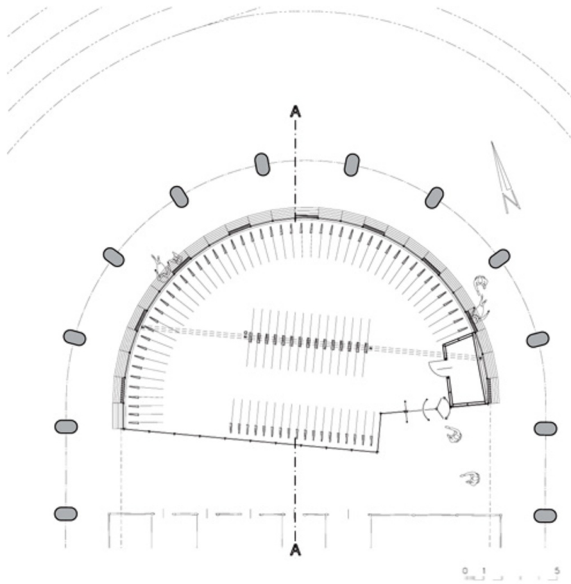
Grundriss
