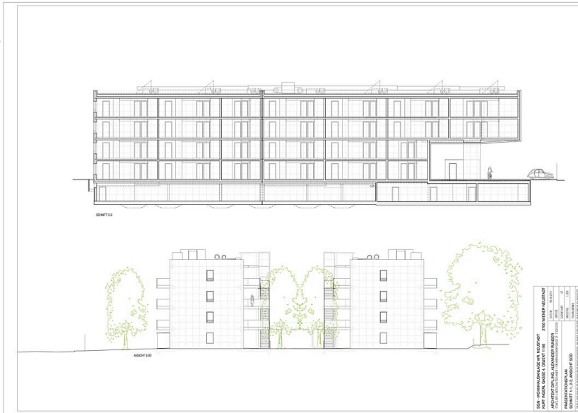
Ansicht Süd, Schnitt 2-2
