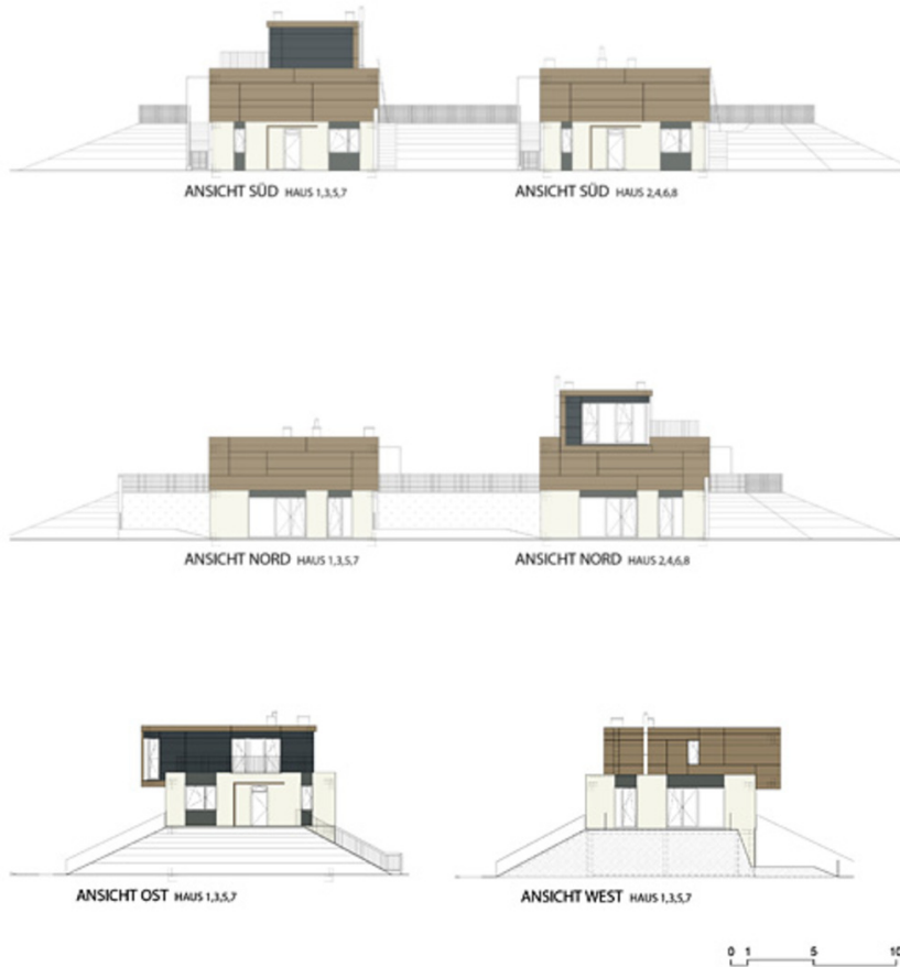
Ansicht
