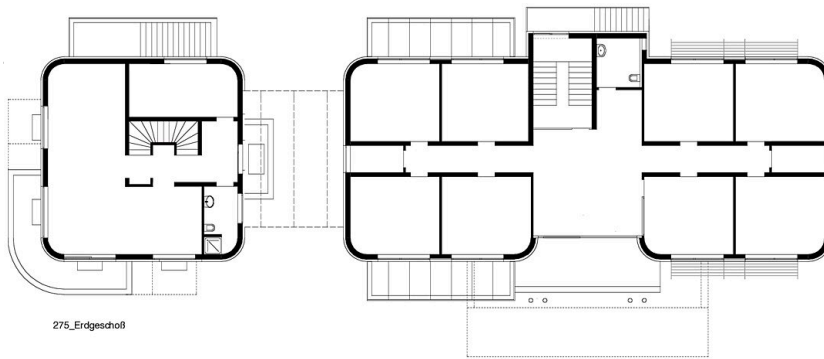
Grundriss Erdgeschoss
