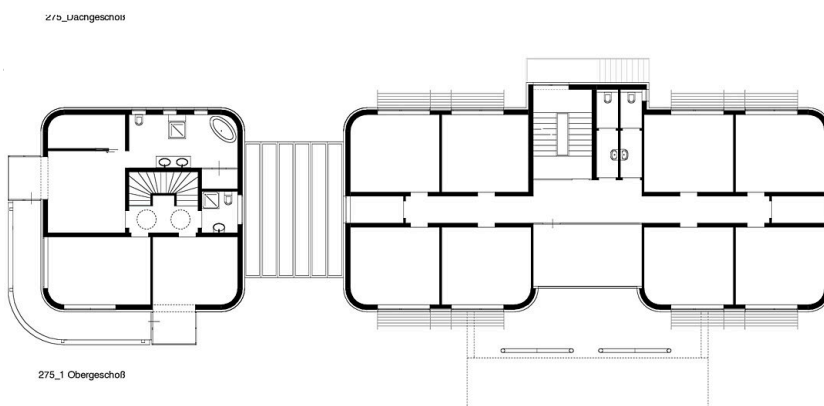
Grundriss Obergeschoss
