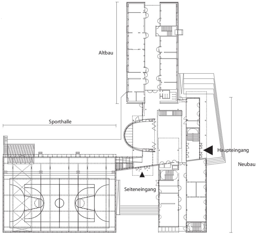
Grundriss Erdgeschoss
