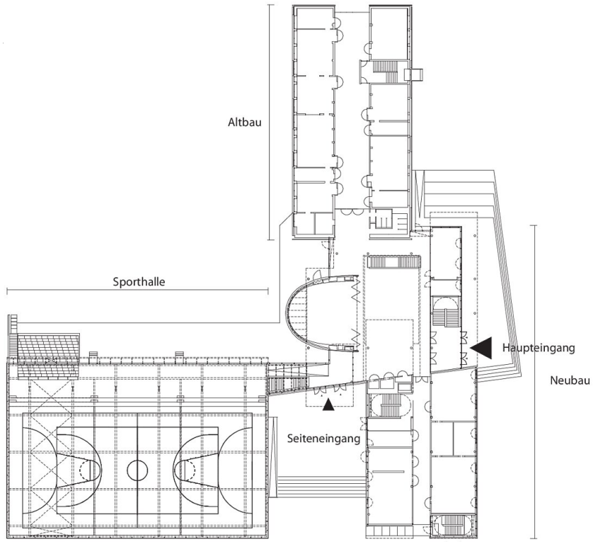
Grundriss Erdgeschoss
