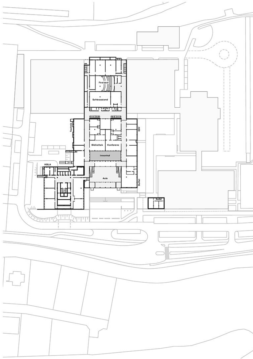
Grundriss Untergeschoss
