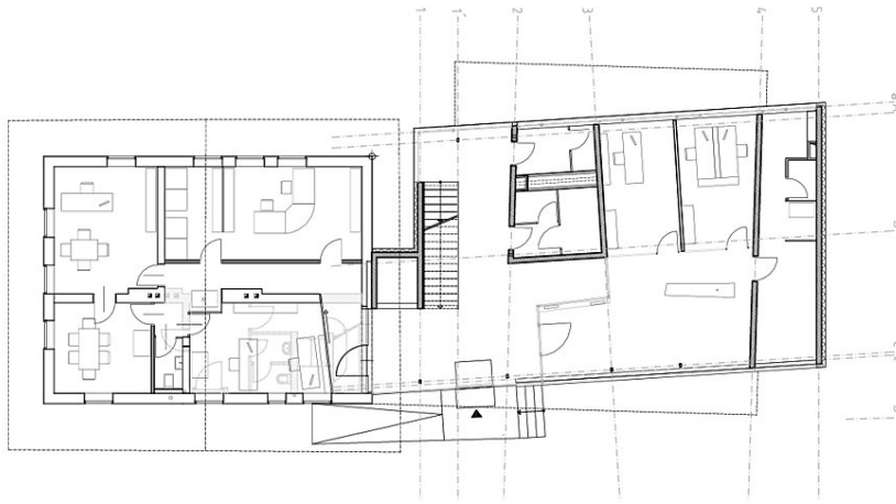
Grundrisse EG + OG
