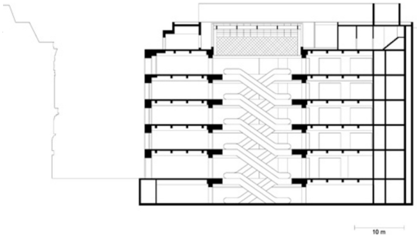
Längsschnitt
