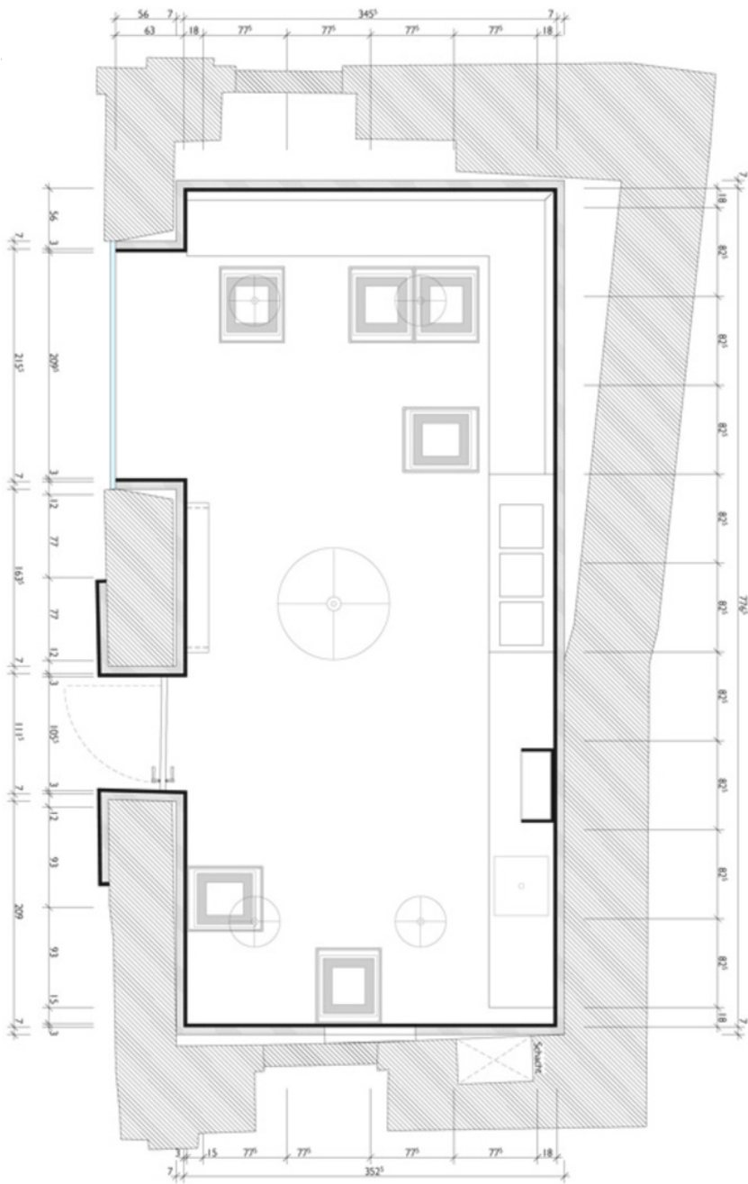
Grundriss
