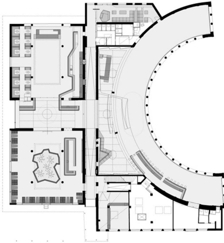
Grundriss
