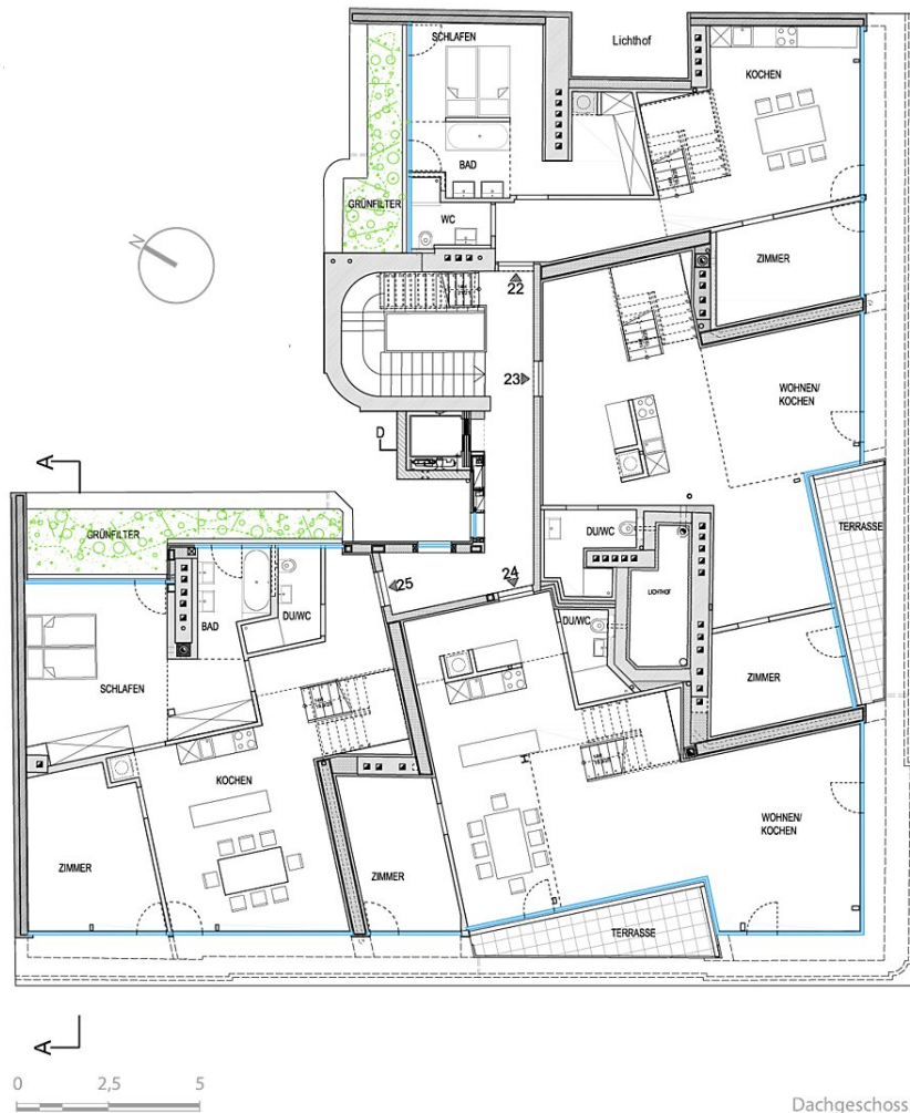
Dachgeschoss 1
