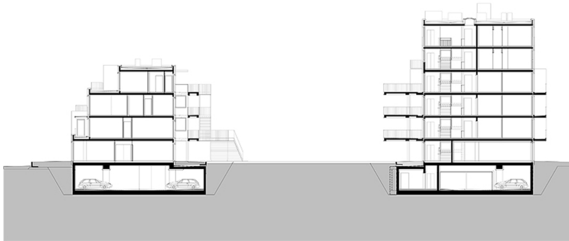
Schnitt 1
