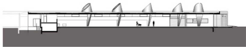
SCHNITT A
