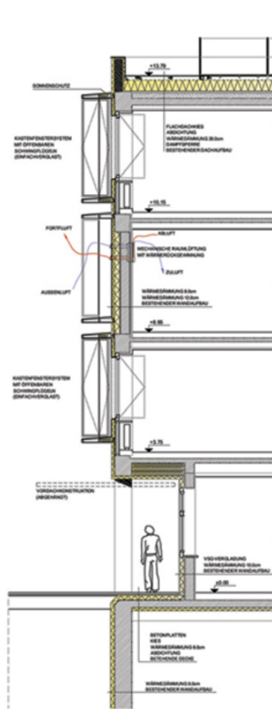
FASSADENSCHNITT | 1:100
