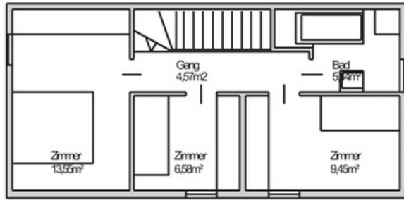
OBERGESCHOSS 39,59m 2
