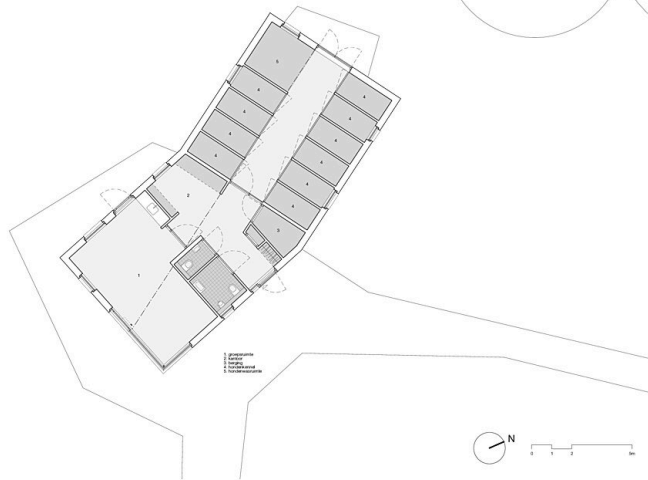
Grundriss Hundezwinger
