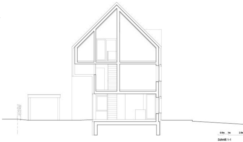
Schnitt
