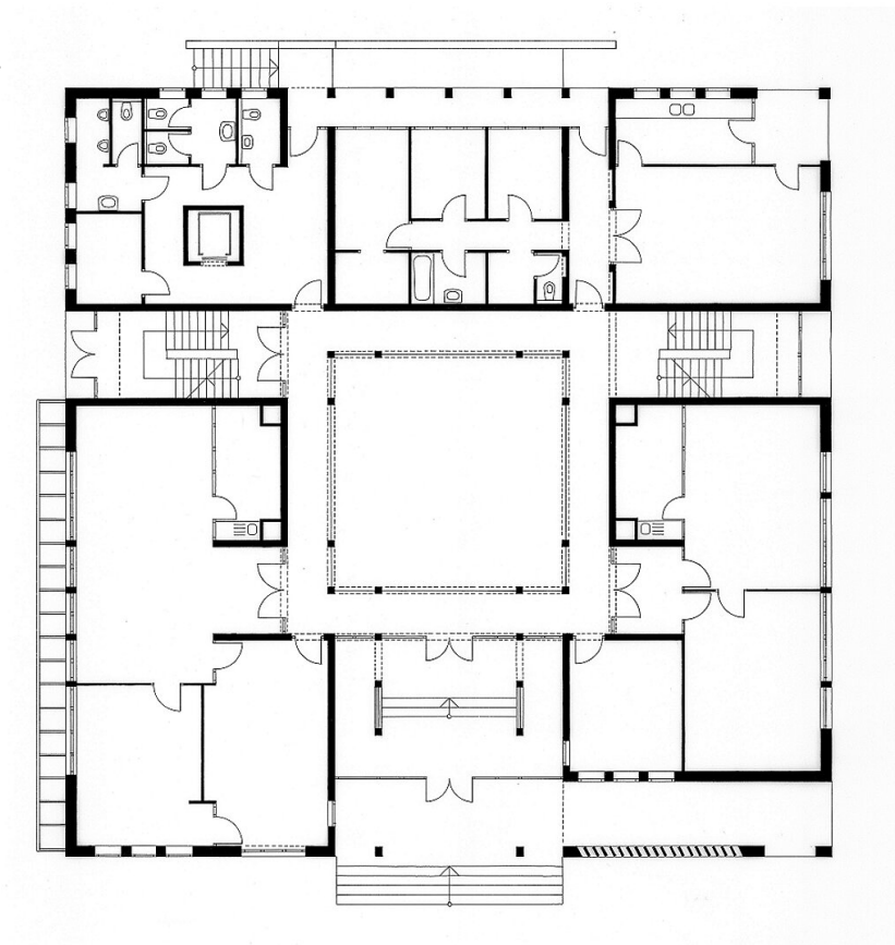
Gemeindehaus Grundriss
