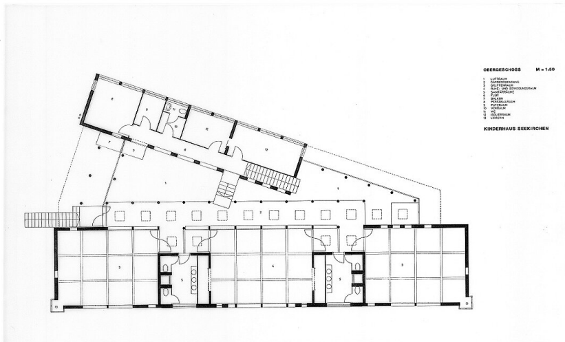
Kinderhaus Obergeschoss
