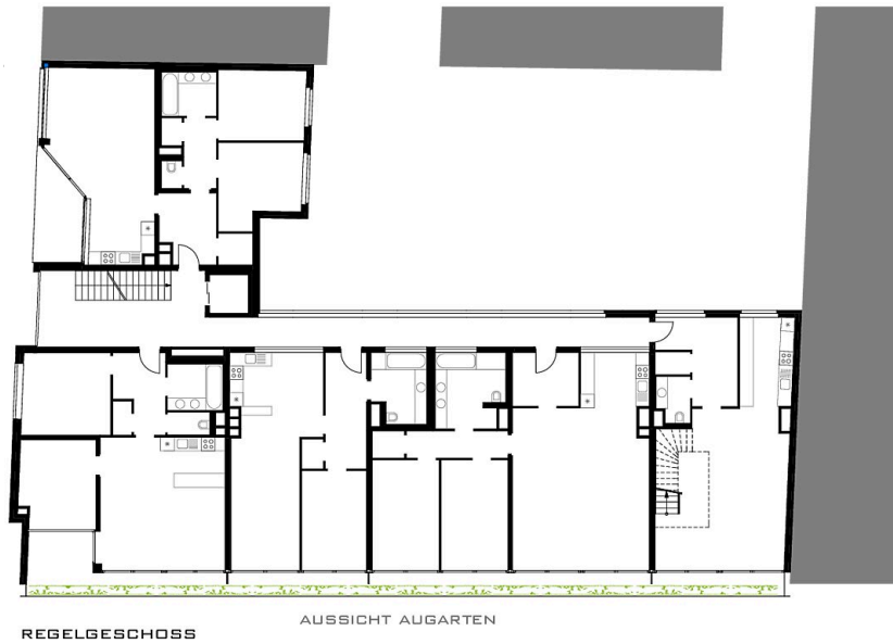
Grundriss Regelgeschoss
