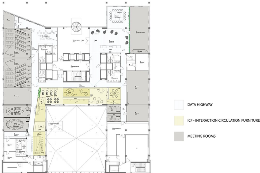
Grundriss Erdgeschoss
