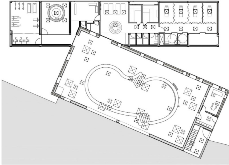
Grundriss
