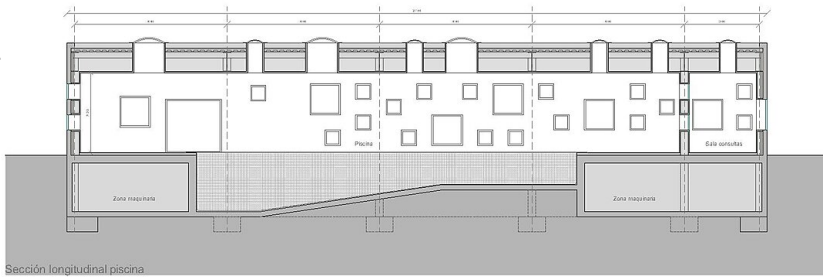
Sección longitudinal piscina
