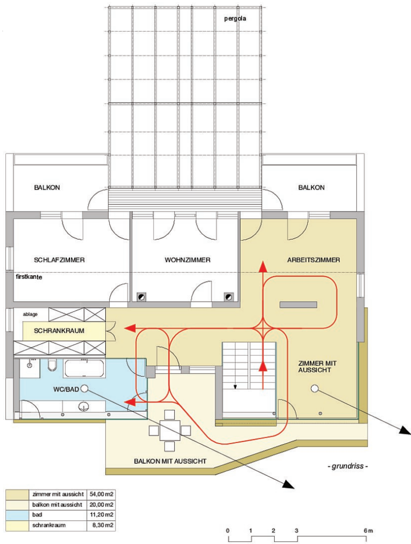
GRUNDRISS, Ansichten
