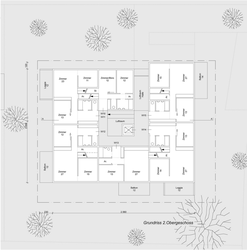
Grundriss OG2
