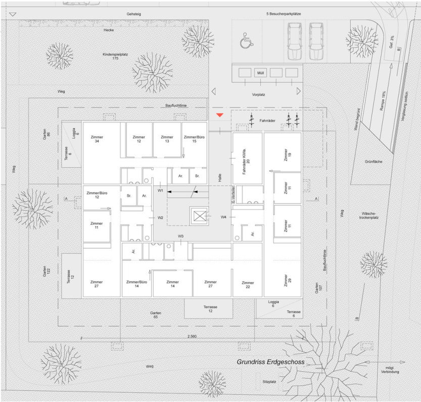
Grundriss EG
