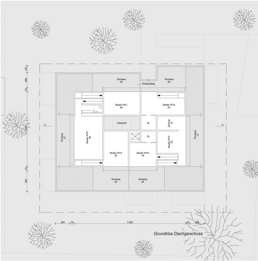
Grundriss DG
